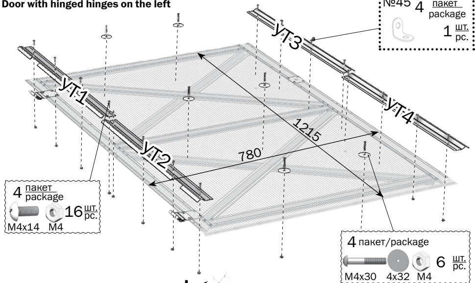
Дверь с петлями навески слева Door with hinged hinges on the left
